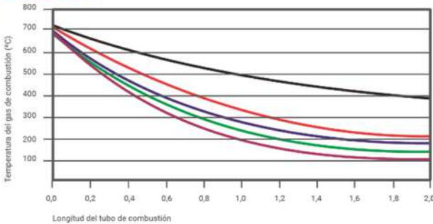
GRÁFICA: CURSO DE LA TEMPERATURA
